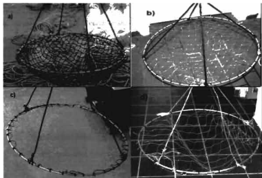
Figura 8.- Aros jaiberos: a) Aro con tamaño de malla de 45 mm, b) Aro con tamaño de malla de 76 mm , c) Aro con tamaño de malla de 101.6 mm y d) Aro con tamaño de malla de 127 mm.
